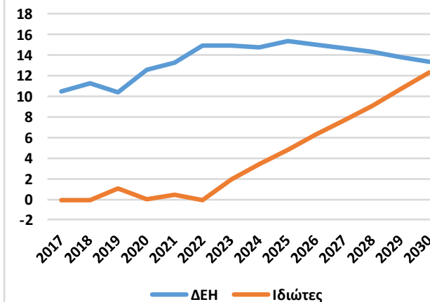
Έλλειμμα (χωρίς ΑΠΕ) στην περίπτωση αποεπένδυσης (TWh)
