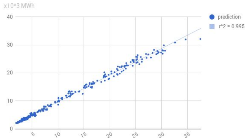
Διάγραμμα διασποράς για εκτίμηση ζήτησης ΦΑ κατά το χρονικό διάστημα 01/06/2016 - 31/10/2017 στο ΣΕΔΔ 'Αθήνα'
