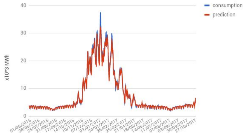
Διάγραμμα ζήτησης / πρόβλεψης ΦΑ στο χρόνο κατά το χρονικό διάστημα 01/06/2016 - 31/10/2017 στο ΣΕΔΔ 'Αθήνα'
